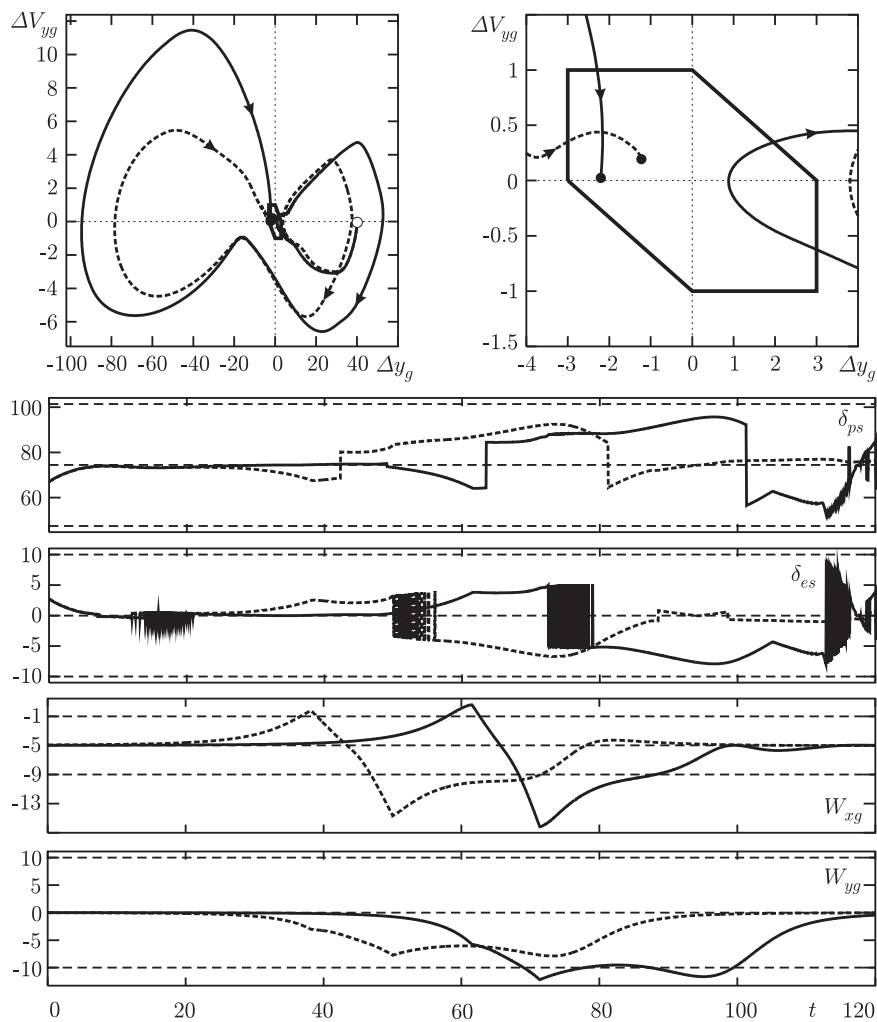
Рис. 2: Моделирование задачи о посадке. Сверху: траектории движения в фазовой плоскости вертикальное отклонение \Delta y_g (м) \times отклонение вертикальной скорости \Delta V_{yg} (м/с). Далее: графики командных управлений по силе тяги \delta_{ps} (град) и рулю высоты \delta_{es} (град); графики продольной W_{xg} (м/с) и вертикальной W_{yg} (м/с) компонент скорости ветра. Пунктир соответствует слабому микровзрыву, сплошная линия — более сильному.
