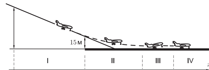
Рис. 1: Процесс посадки самолета. В работе рассматривается I этап — снижение по глиссаде до пролета торца ВПП. Далее следуют: II этап — выравнивание, III этап — пробег на колесах главной стойки шасси, IV этап — пробег на всех колесах.
