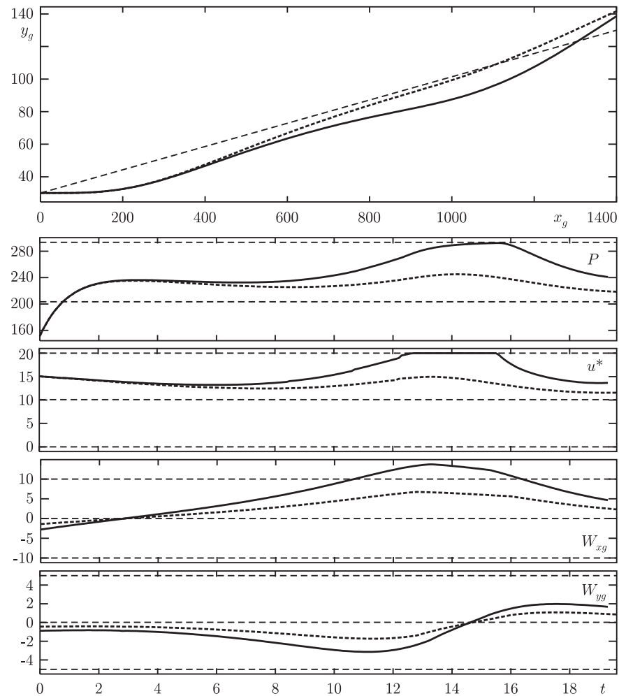
Рис. 4: Моделирование задачи о преодолении препятствия по высоте. Сверху: график высоты (м). Далее: графики силы тяги P (Н), целевого угла тангажа u^* (град), продольной W_{xg} (м/с) и вертикальной W_{yg} (м/с) компонент скорости ветра.
